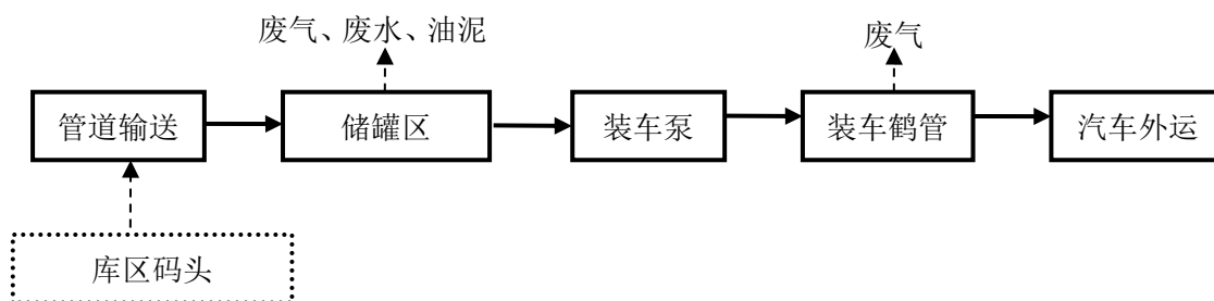
图 2.4-1 原油进出库流程及产污环节图
