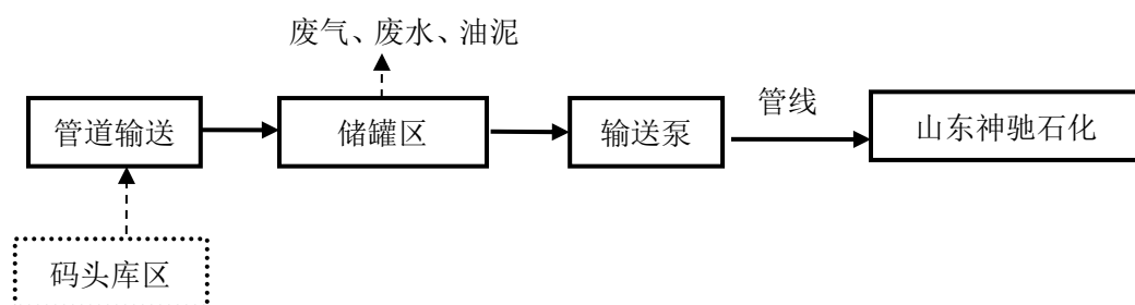
图 2.4-2 渣油进出库流程及产污环节图
