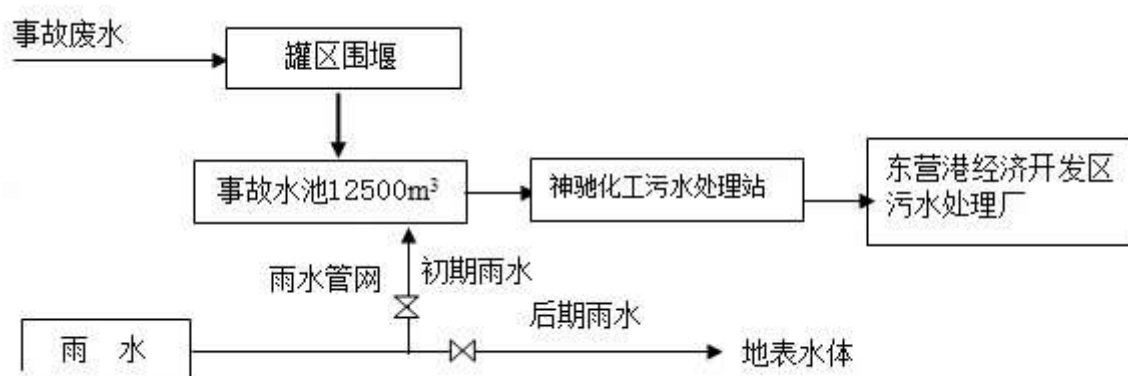
图 3.4-1 项目初期雨水和事故废水收集导排系统示意图
