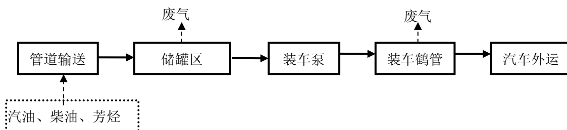
图 2.4-3 汽油、柴油、芳烃进出库流程及产污环节图
